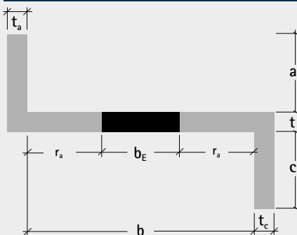
TIPO DE SECCIÓN TRANSVERSAL Z
