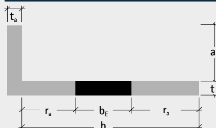
TIPO DE SECCIÓN TRANSVERSAL L
