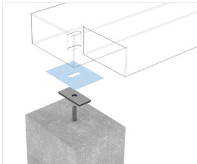
Ejecución del taladro / orificio oblongo
